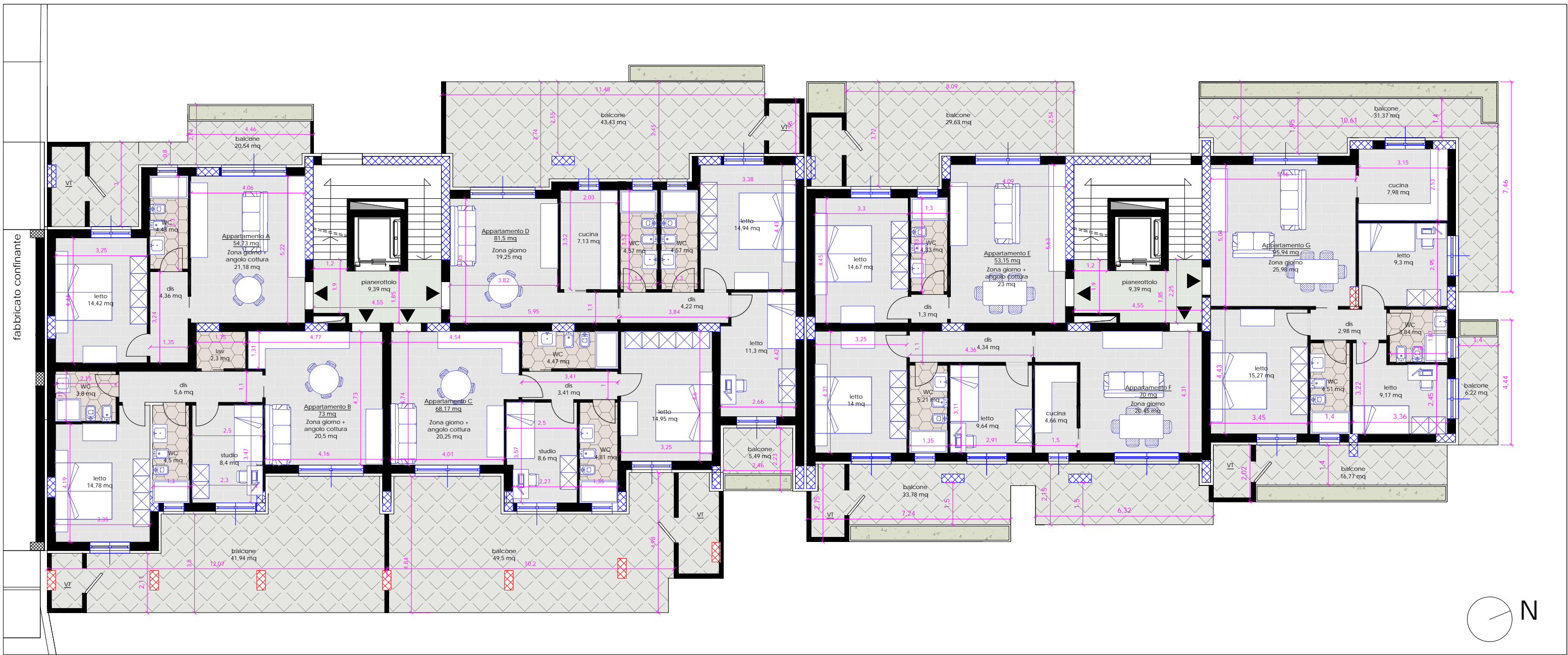
PLANIMETRIA PIANO SECONDO - QUARTO E SESTO
